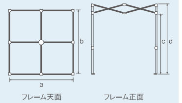
軸組図
